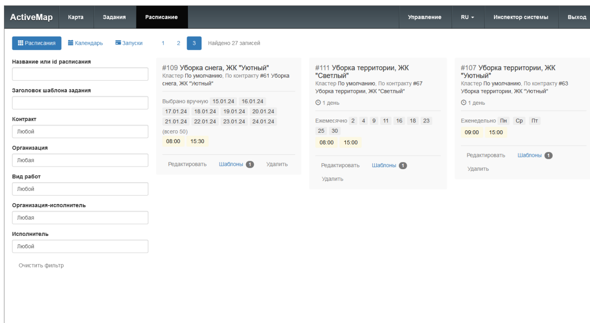
Рис. 2.51: Карточки расписаний
