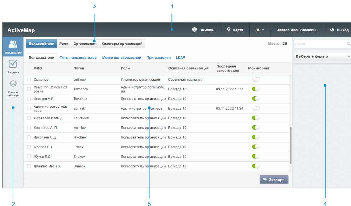
Рис. 2.55: Модуль управления
