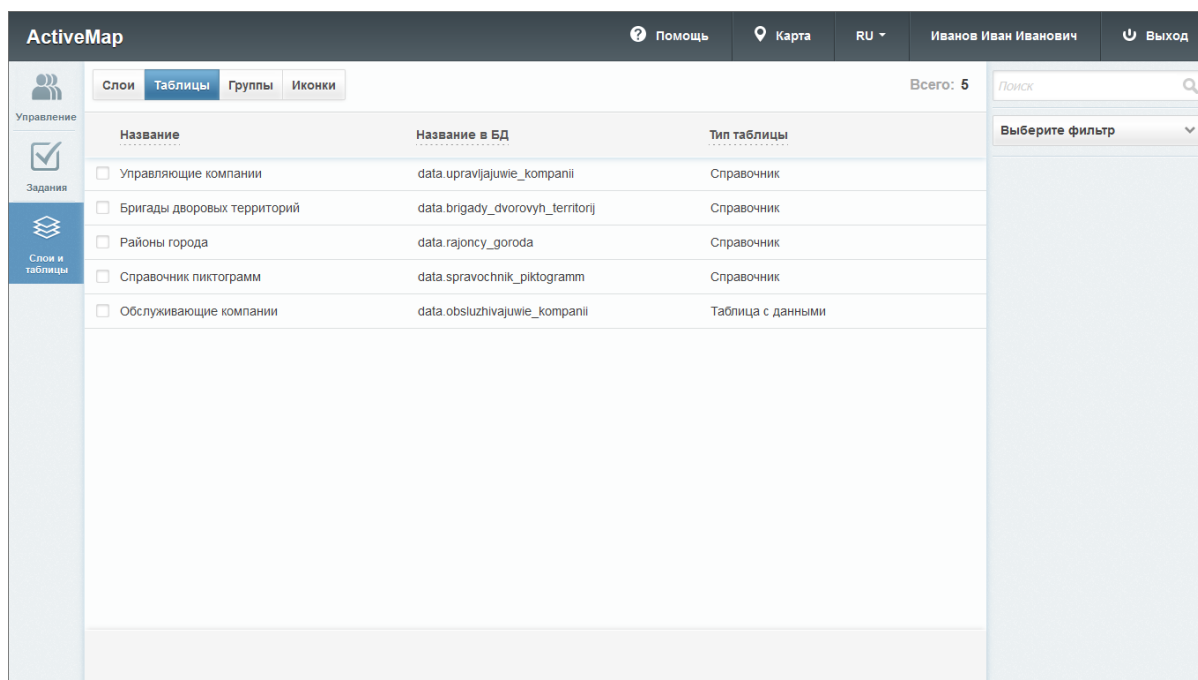
Рис. 2.89: Вкладка «Таблицы»
