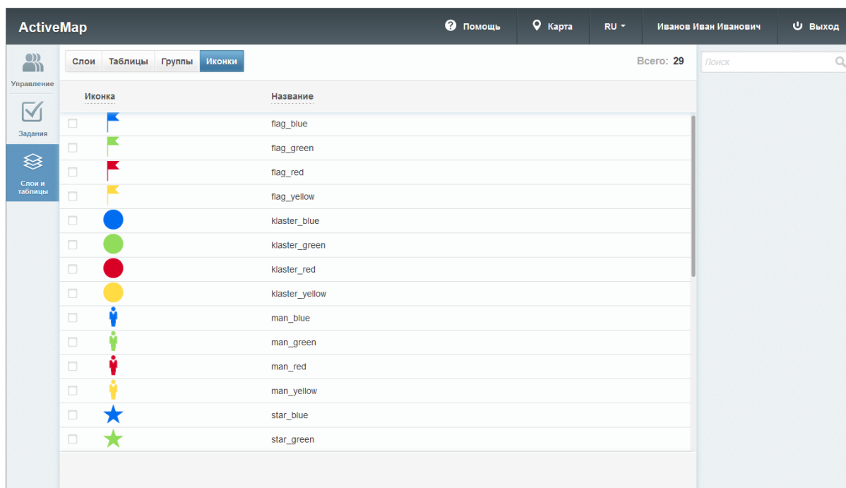
Рис. 2.91: Вкладка «Иконки»
